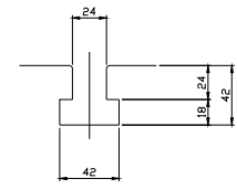
T홈부 상세 (S=1:3)
